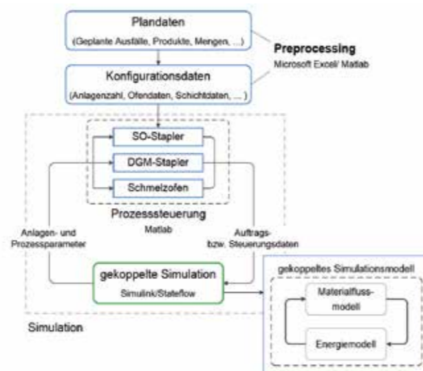
Aufbau der Simulation
