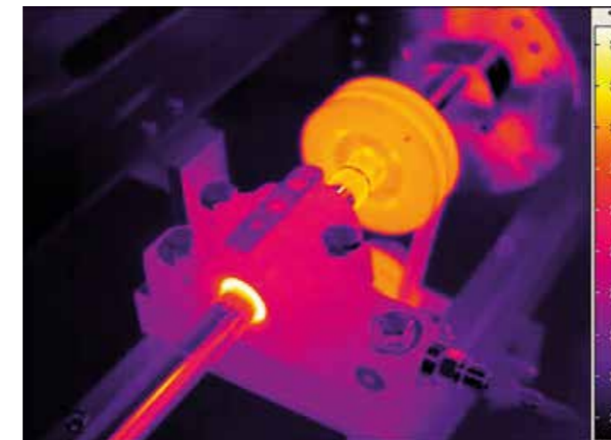
Thermografieaufnahme Wellenlagerung: Thermografie macht die Erwärmung durch betriebsbedingte Reibung sichtbar
